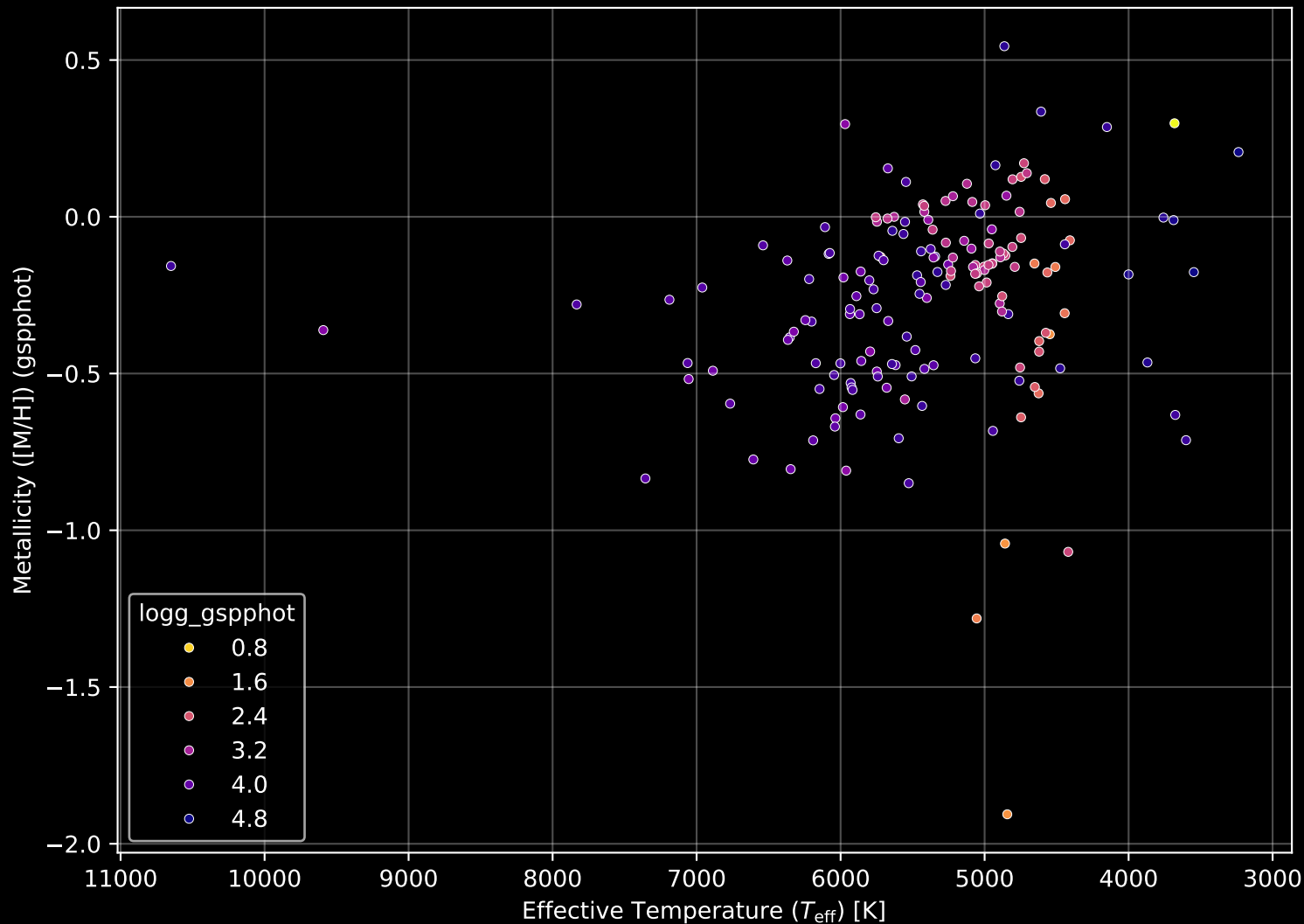
APOGEE DR17 Field: [279-19-O_TESS] Stellar Population Parameters (n= 171)
